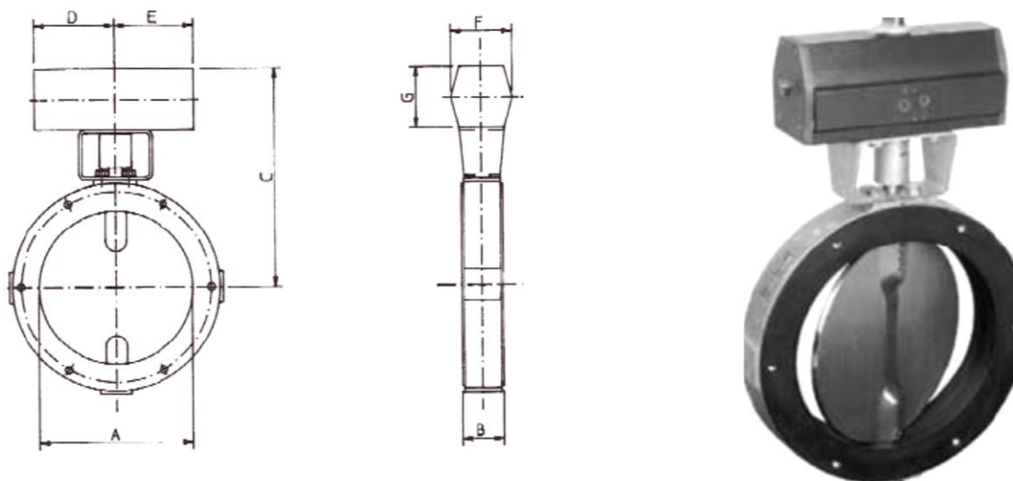
Vridspjällsventil med vriddon
