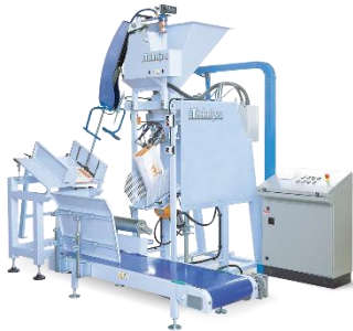
Gravimetrisk fyllning.
